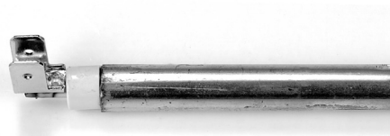
Doppel-Flachstecker, 90° Winkel.
