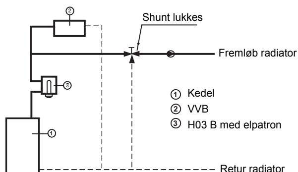
Principskema for kedel med ekstern varmtvandsbeholder
