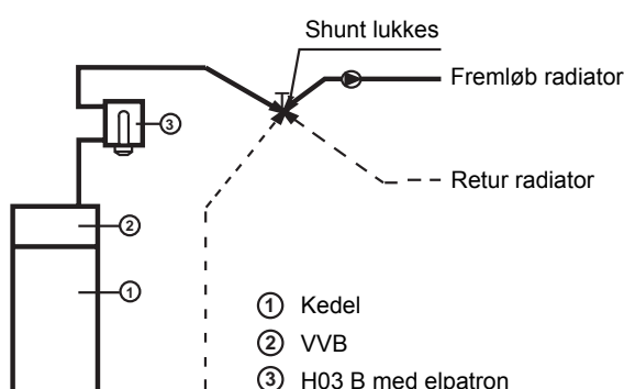
Principskema for kedel med indbygget varmtvandsbeholder
